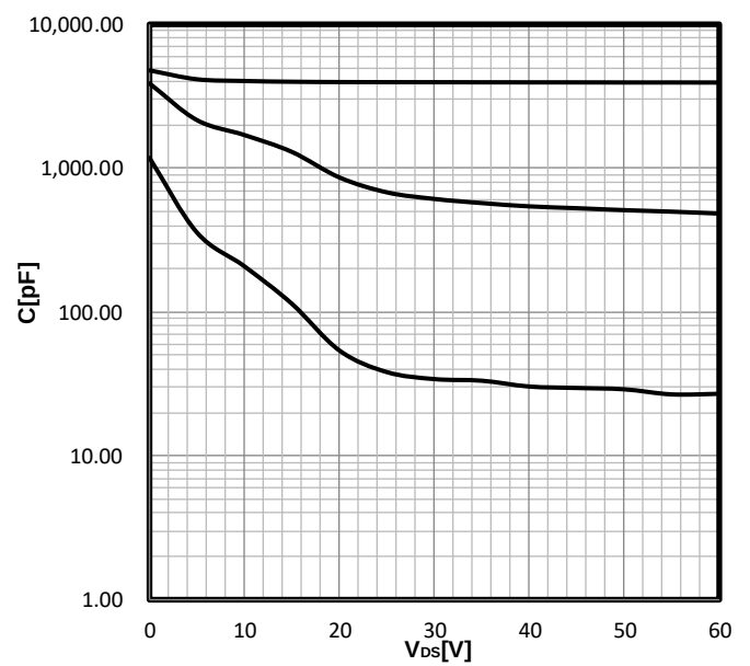
Typ. capacitances
