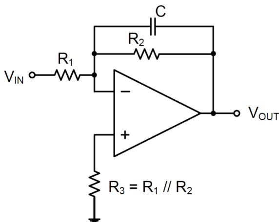
图6，低通滤波器
