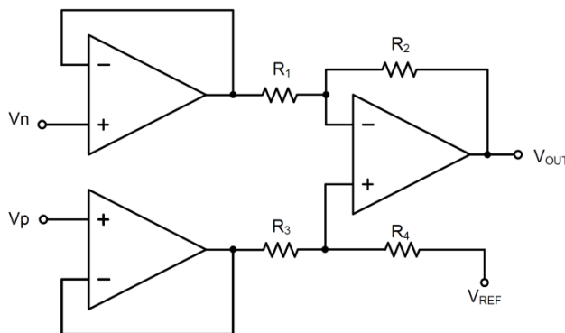
图5，精密放大电路
