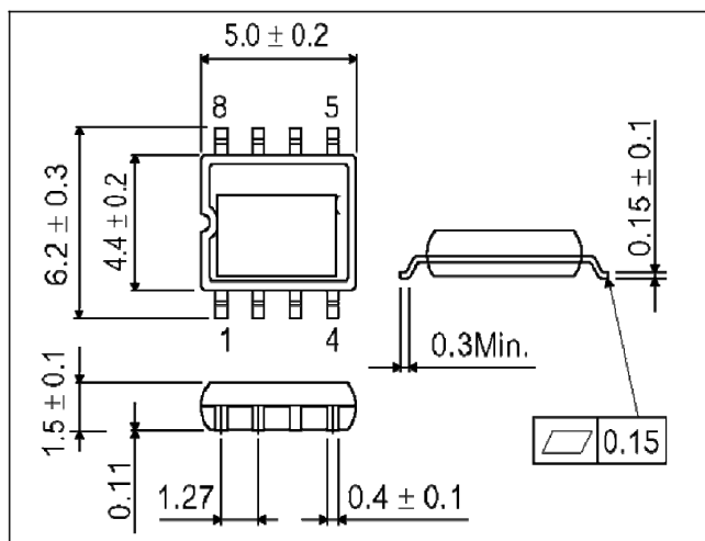
SOP8
