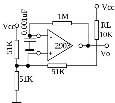
方波振荡器
